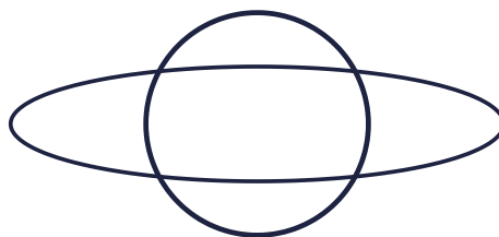
6. どせい
