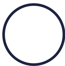
2. きんせい
