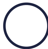
4. かせい
